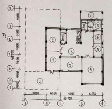
План на висоті +4,500 м М 1:400
