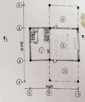
План на висоті +7,500 м М 1:300
