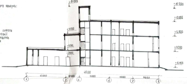
Розріз 1-1 М 1:200
