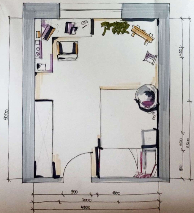
ВАРІАНТ №1 ПЛАН М 1:25
